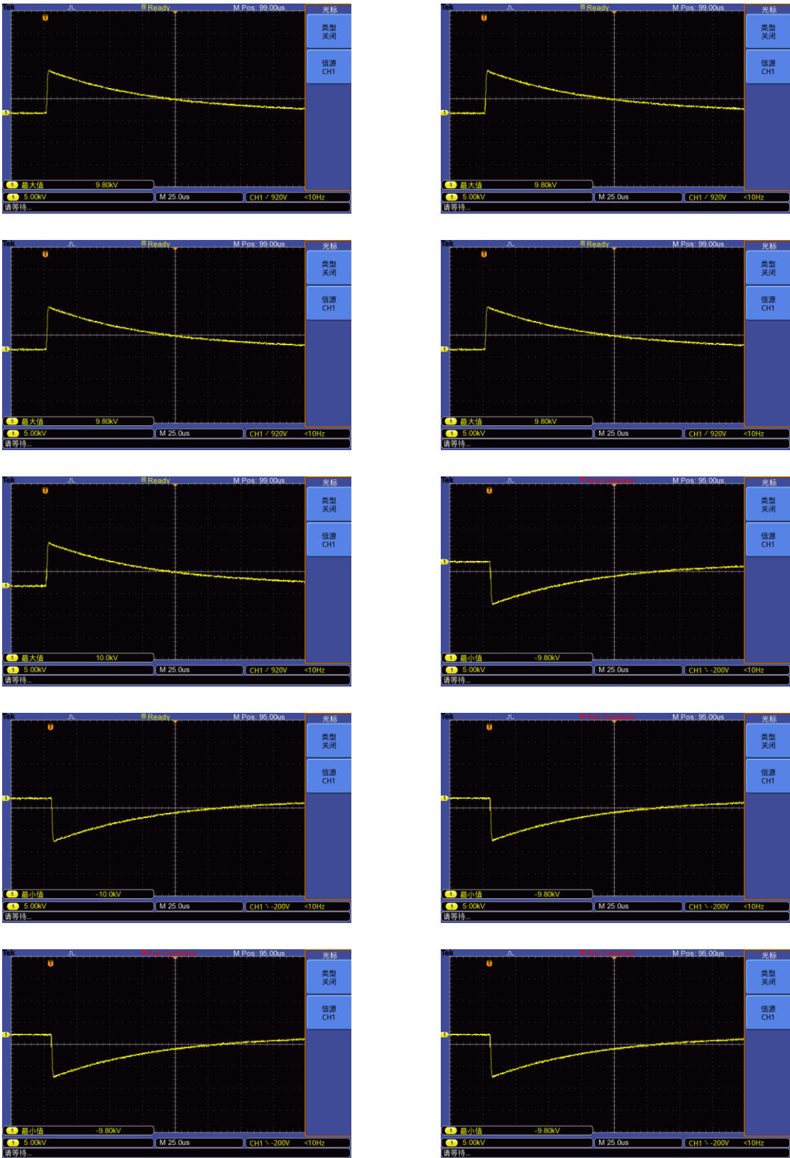
冲击耐受电压试验示波图（9. 80kV）
