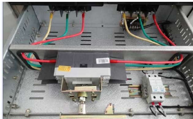
出线 5 抽屉照片
