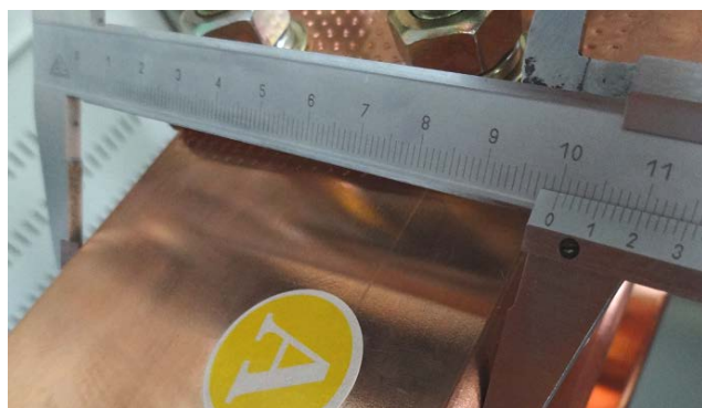
水平母排宽度照片
