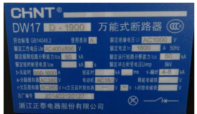
主断路器铭牌照片
