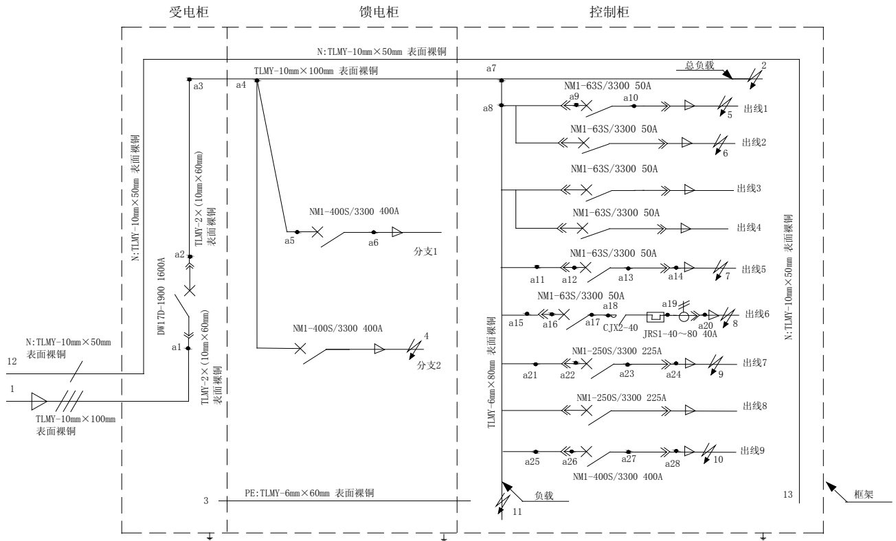
温升、短路点示意图 F1
