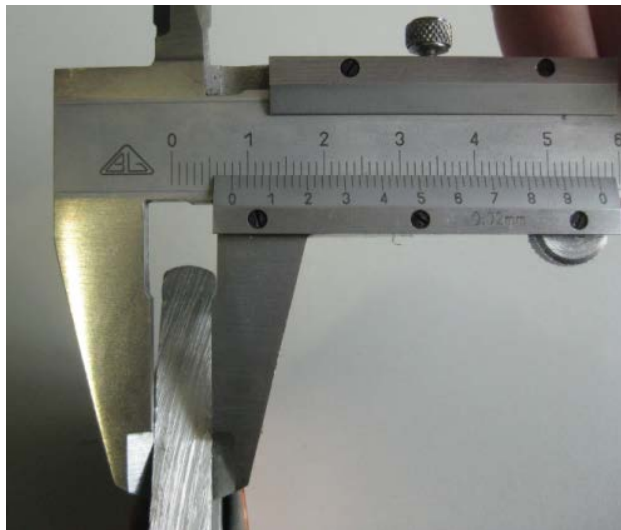
TLMY-10mm×60mm 铝层厚度 (8.00mm) 照片
