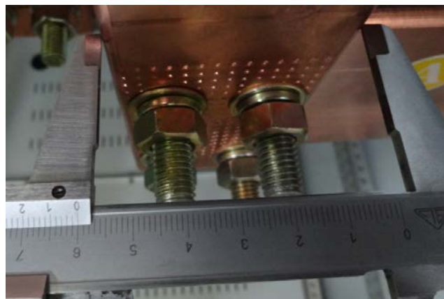
主开关进出线母排宽度照片
