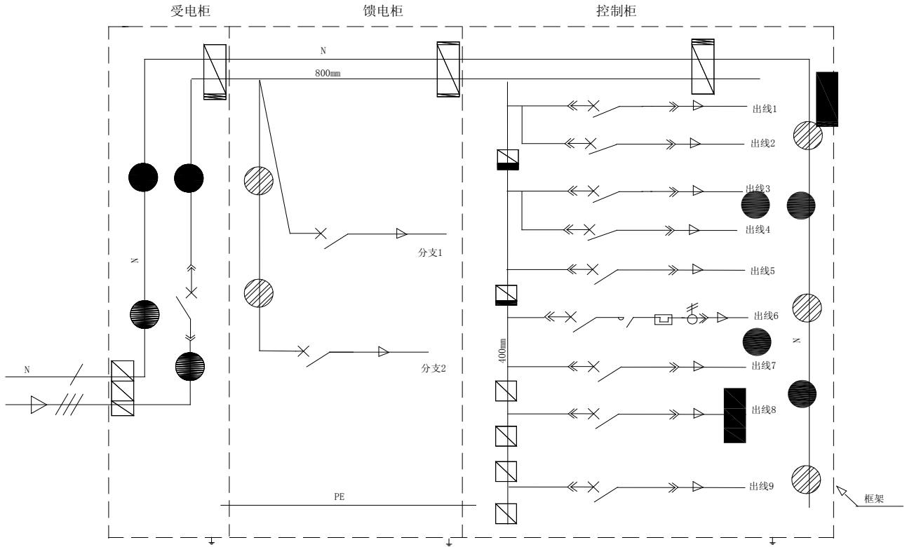
母排绝缘支撑件及绝缘夹板的安装布置图 F2
