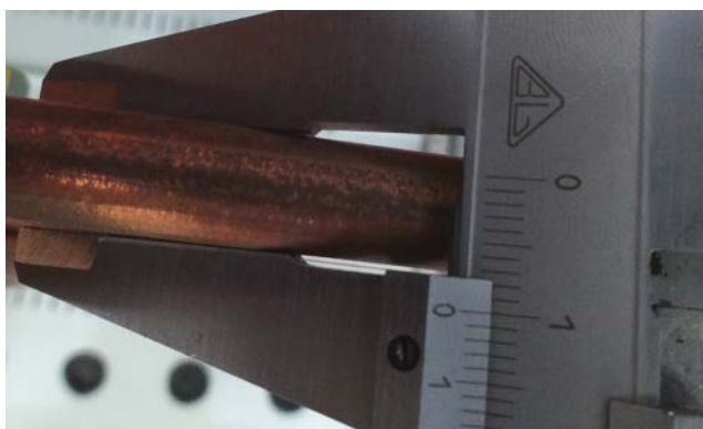
水平母排厚度照片
